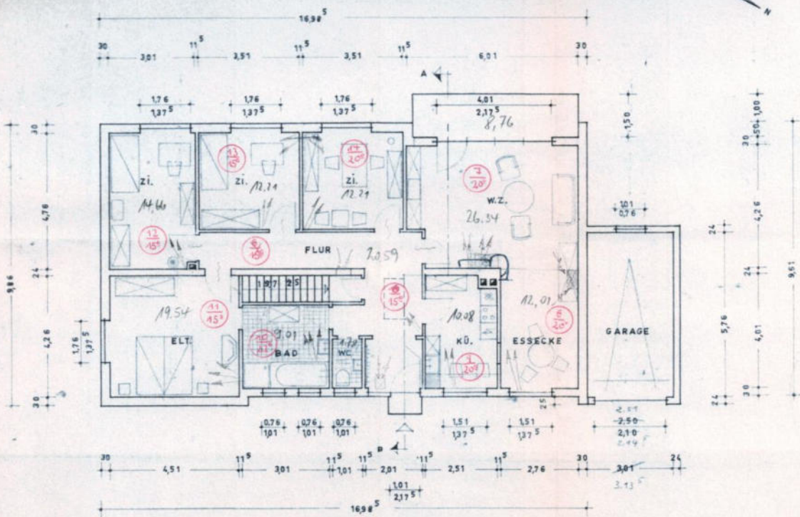
ERDGESCHOSS M. 1:100
