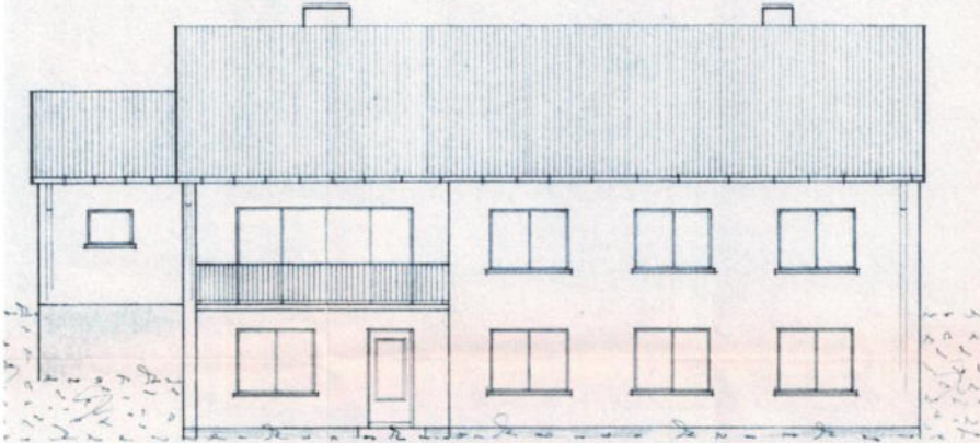
ANSICHT VON SÜD - WEST
