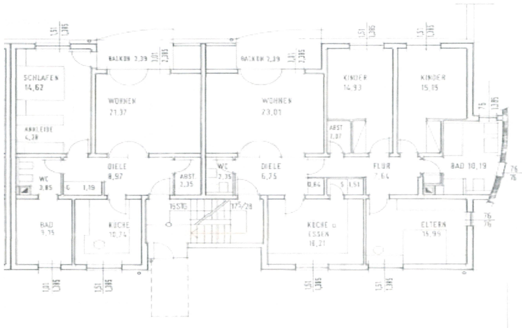
Erdgeschoss und 1. OG
